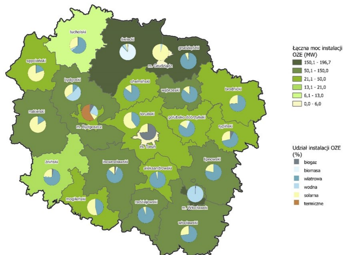
Instalacje OZE na terenie powiatów województwa kujawsko-pomorskiego bez mikroinstalacji prosumenckich według stanu na 30 czerwca 2023 r.
