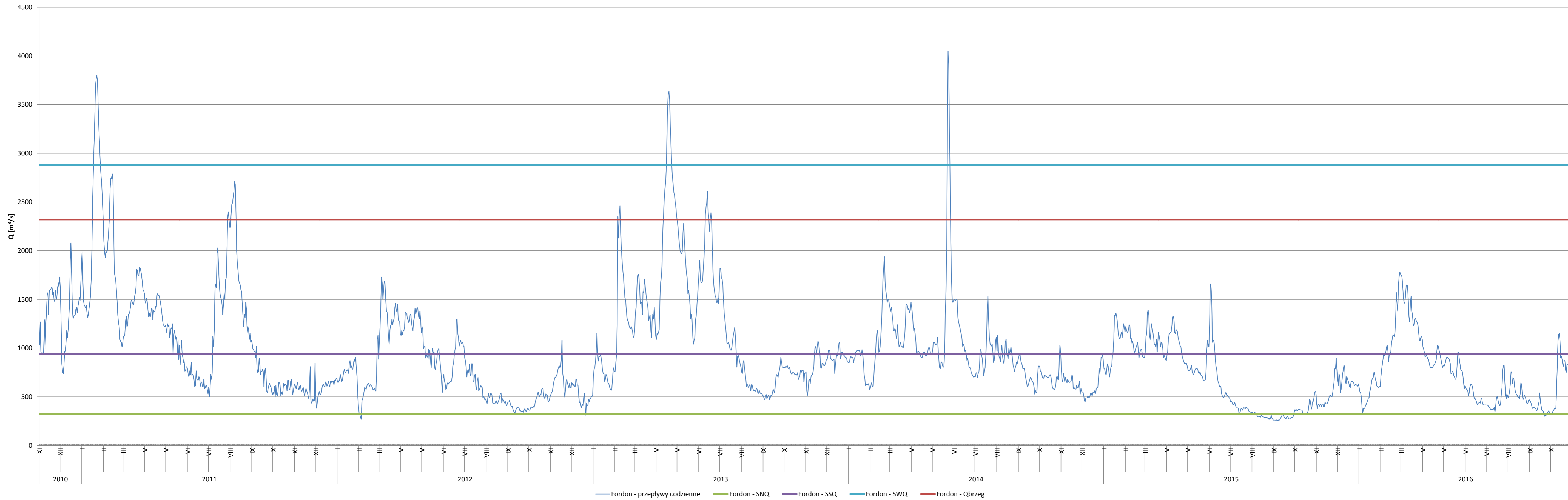
Hydrogram przepływów dla wodowskazu Fordon (2011-2016r.)
